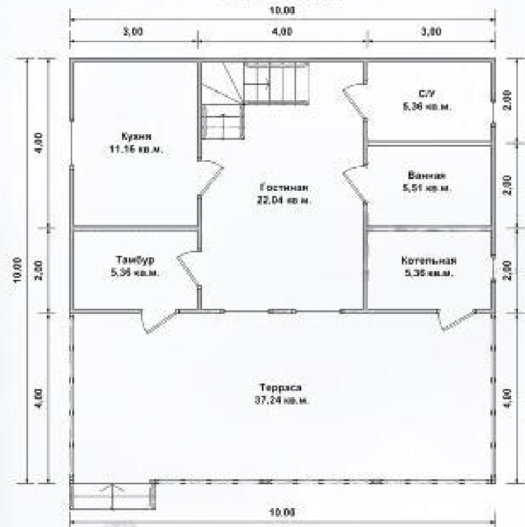
План 1-й этаж
