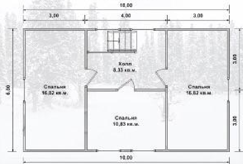
План 2-й этаж
